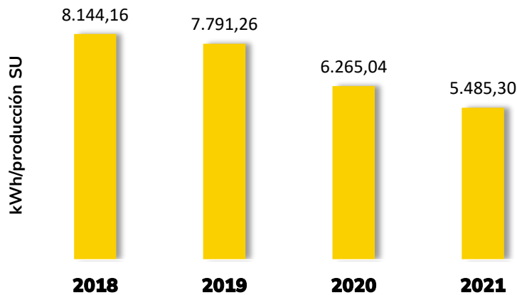
Ilustración 15. Evolución del consumo de energía eléctrica en relación con la producción del sector uniformidad en la lavandería de ILUNION en Valladolid
