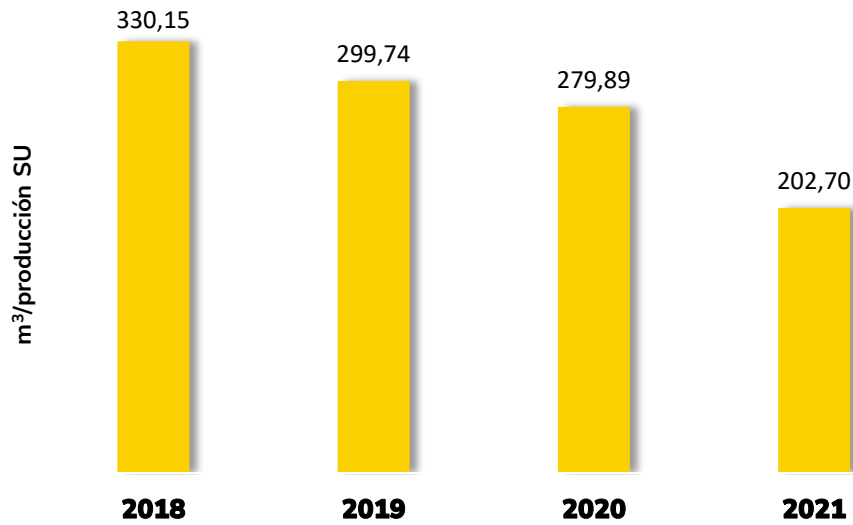
Ilustración 11. Evolución del consumo de agua en relación con la producción del sector uniformidad en la lavandería de ILUNION en Valladolid
