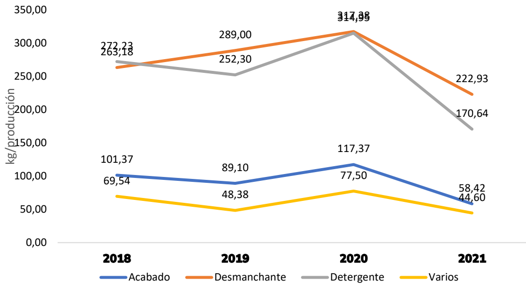
Ilustración 29. Evolución del consumo de materiales en relación con la producción Global en la lavandería de ILUNION en Valladolid
