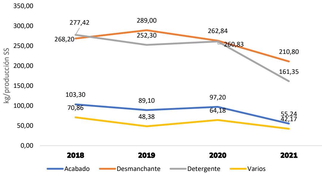
Ilustración 30. Evolución del consumo de materiales en relación con la producción del sector sanitario en la lavandería de ILUNION en Valladolid
