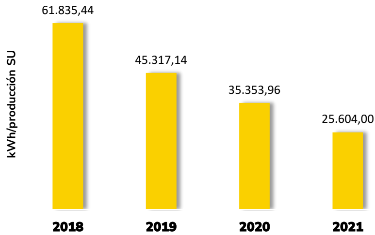
Ilustración 19. Evolución del consumo de GN en relación con la producción del sector uniformidad en la lavandería de ILUNION en Valladolid
