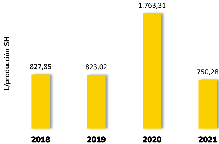
Ilustración 24. Evolución del consumo de combustible asociado a la flota de vehículos en relación con la producción en la lavandería de ILUNION en Valladolid (Sector Hotelero)
