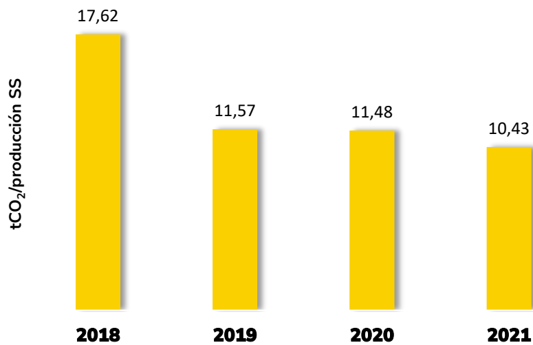
Ilustración 38. Evolución de las emisiones de CO 2 en el centro de ILUNION en Valladolid en relación con la producción del sector sanitario
